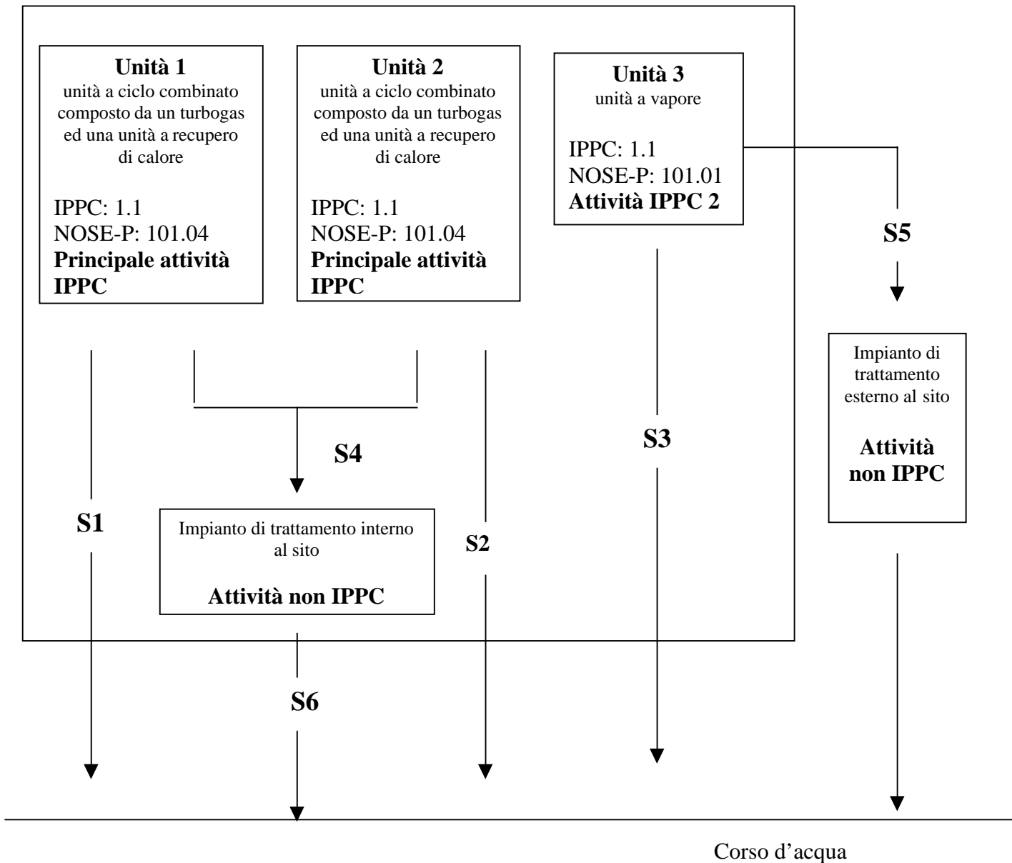
Fig. 3 – Complesso IPPC
